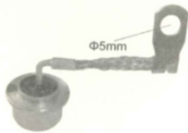
FD91E-35P3 (+) / FD91E-35N3 (-)
